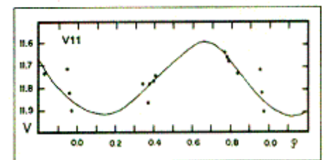
Curva de brillo de la variable 11 de M 13. (F. Violat)
