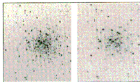
Bajada aparente de L222, debida al polvo en suspensión. (F. Violat)
