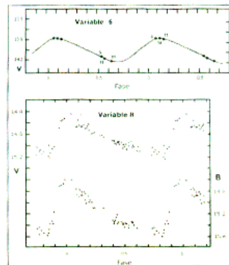
Curvas de luz de las variables 6 y 8 de M 13. (F. Violat)
