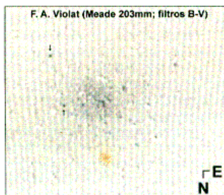
M13, captada con filtro B-v. (F. Violat)
