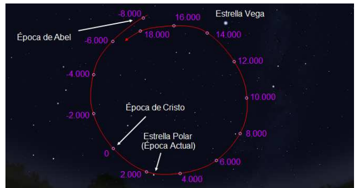
Desplazamiento del polo norte celeste en un ciclo de precesión
