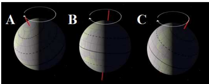
Movimiento de Precesión
